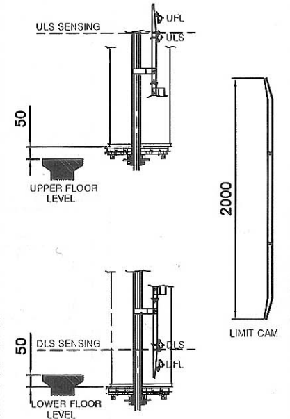
*LIMIT SWITCH SETTING LAYOUT* (NONE SCALE)
