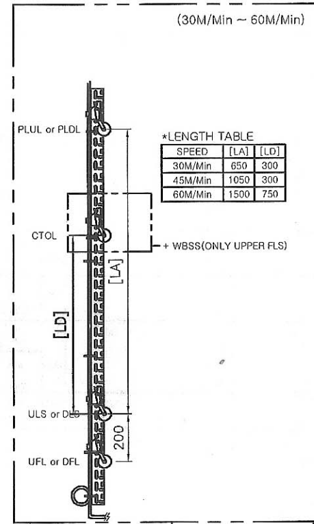
*LIMIT SWITCH SETTING LAYOUT* (NONE SCALE)
